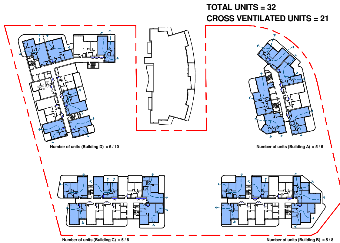
4 CROSS VENTILATION -LEVEL 9 1 : 500
