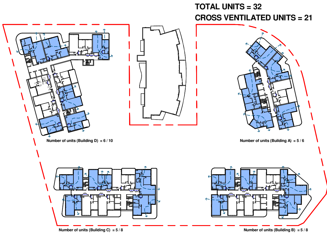
3 CROSS VENTILATION -LEVEL 8 1 : 500
