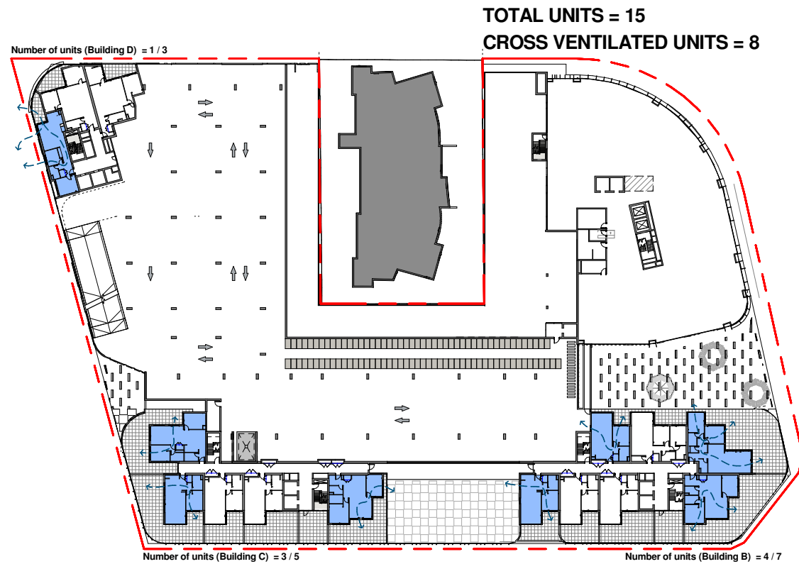
1 CROSS VENTILATION -LEVEL 2 1 : 500
