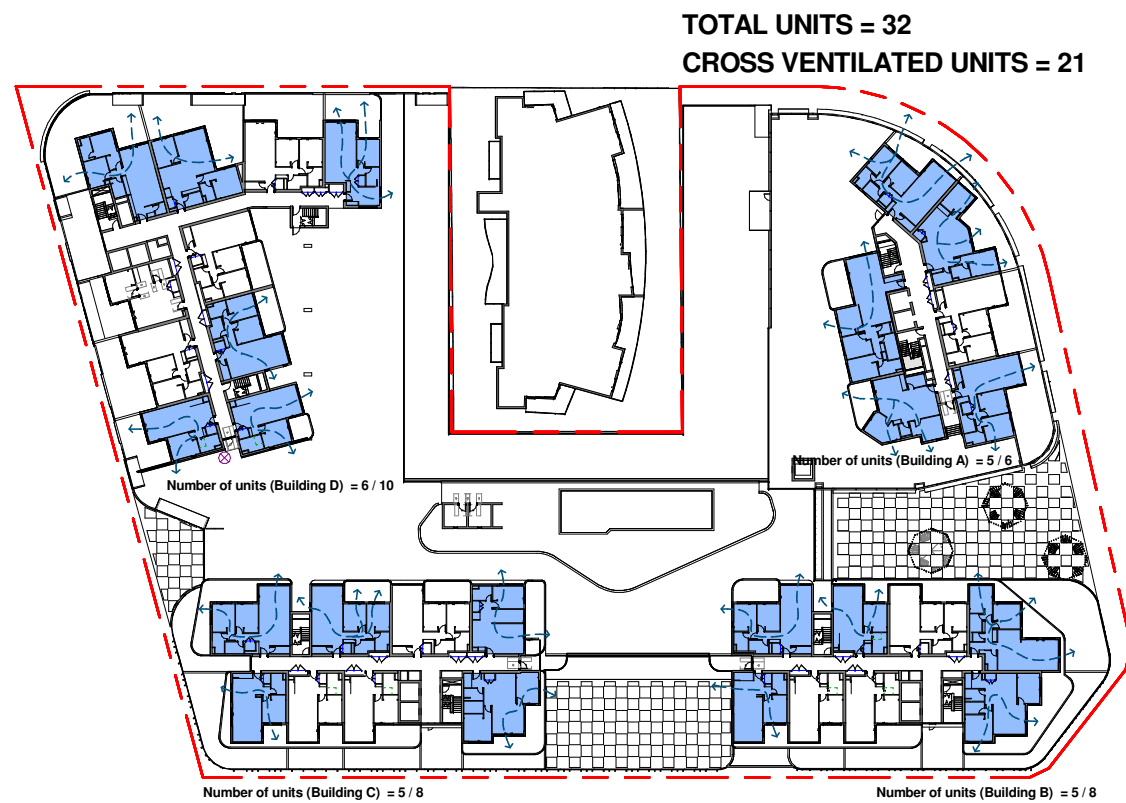
4 CROSS VENTILATION -LEVEL 4 1 : 500
