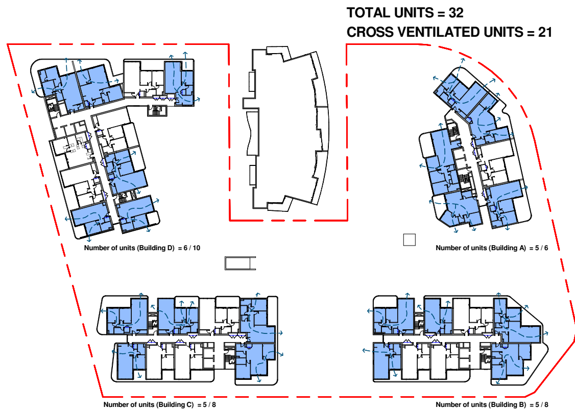
2 CROSS VENTILATION -LEVEL 5 1 : 500
