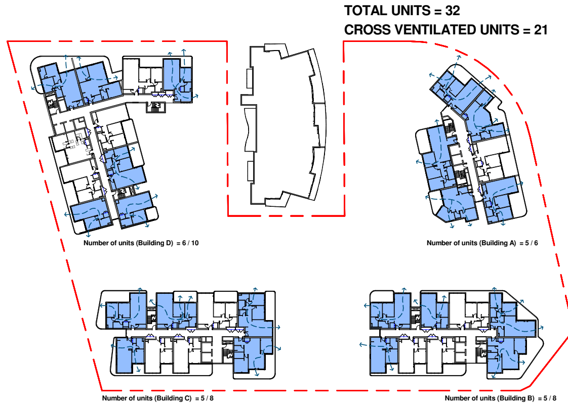
2 CROSS VENTILATION -LEVEL 7 1 : 500
